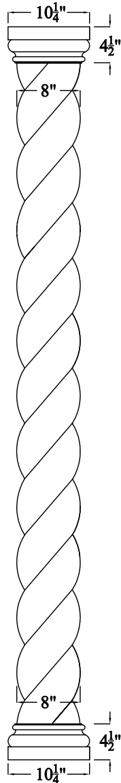
COL8S
