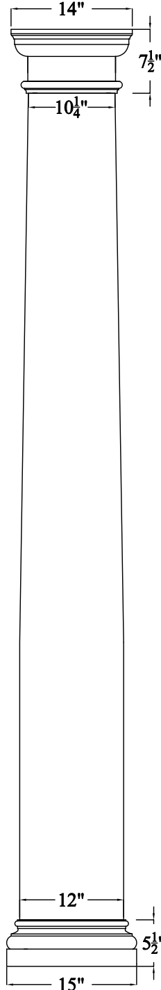
COL12B
