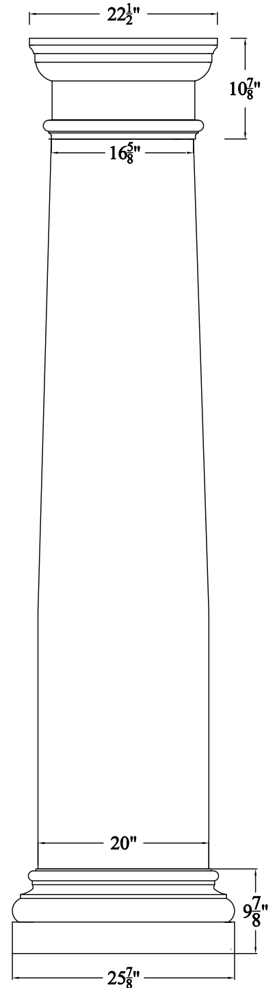
COL20B
